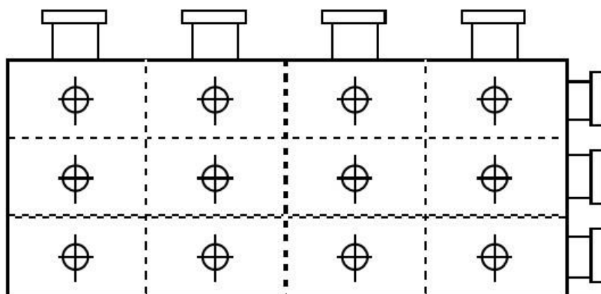
Hình 4: Phân bố 12 điểm hút mẫu đối với ống khối hình chữ nhật
