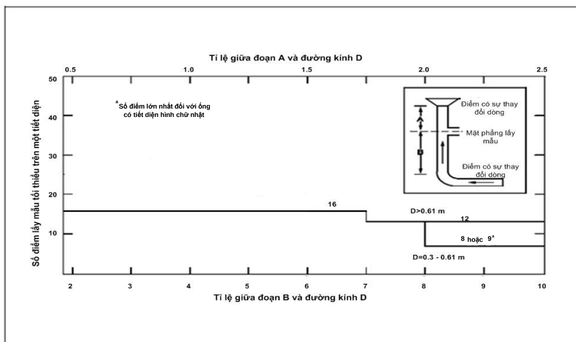
Hình 2. Đồ thị lựa chọn số điểm hút mẫu tối thiểu theo phương ngang
